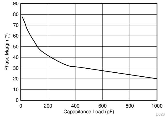
图 7-26. Phase Margin vs Capacitive Load
