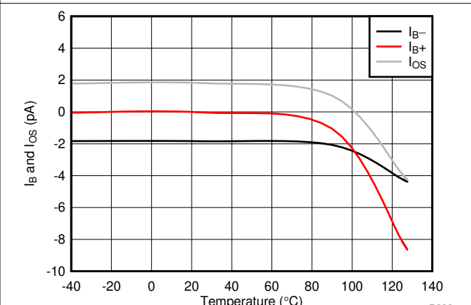
图 7-6. I_B and I_{OS} vs Temperature
