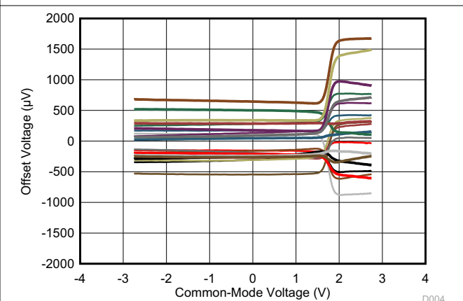
图 7-4. Offset Voltage vs Common-Mode
