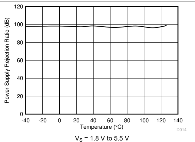
图 7-14. DC PSRR vs Temperature
